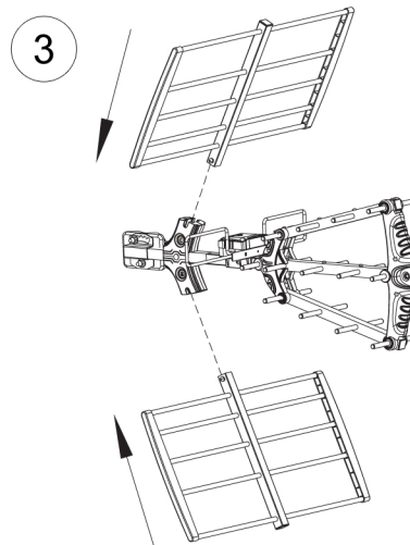
Przymocuj poprzeczne skrzydła anteny
