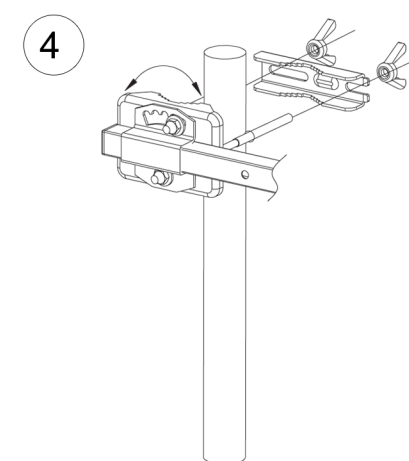
Przymocuj antenę do masztu przy pomocy śrub (załączonych do opakowania) jak pokazano na rysunku
